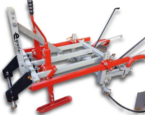
exemple d'un cadre 100% mécanique avec mancherons
