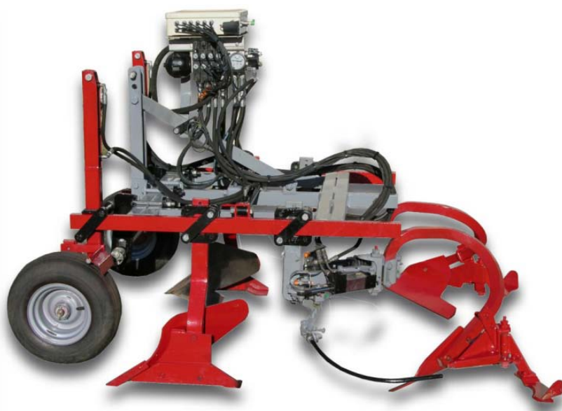
MS-330-TH sur cadre avec charrues
