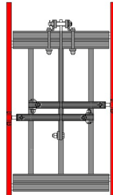
les cadres doubles
